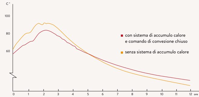
Questo grafico rappresenta la dispersione di calore dopo l'ultima carica di legna.
