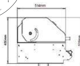
DIMENSIONI GENERALI
