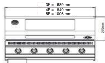
DIMENSIONI GENERALI
