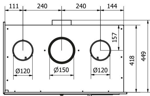
B-B (1 : 8)
