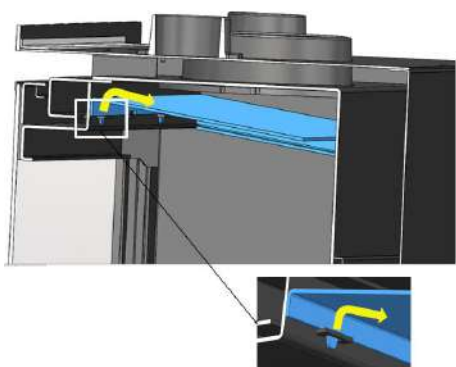
Figura n°23 - Smontaggio del deflettore superiore in acciaio
