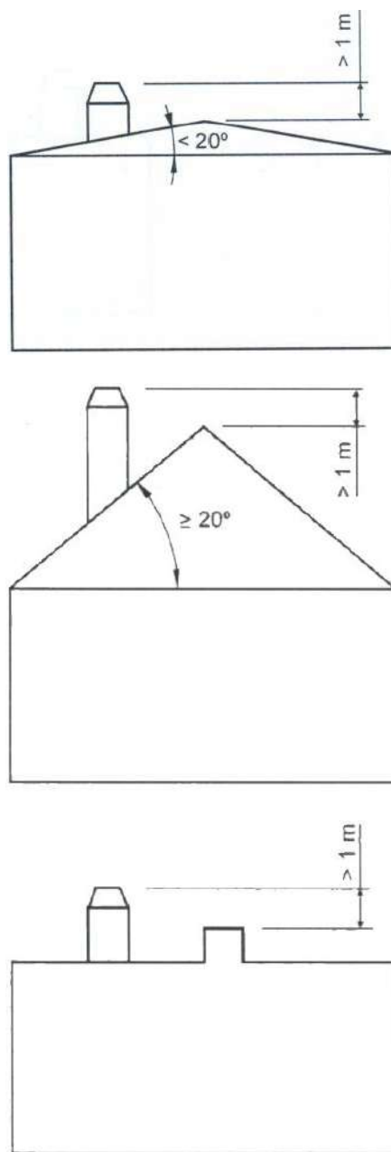
Figura n°17 - Distanza tra la finitura e il colmo del tetto
