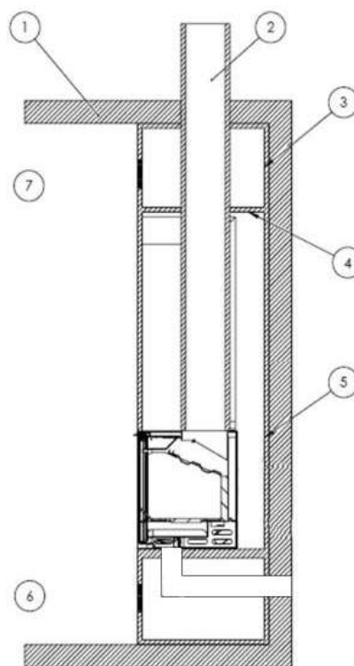
Figura n°5 - Schema interno del rivestimento
