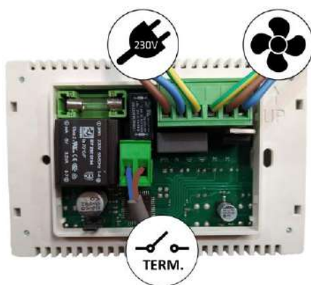
Figura n°16 - Collegamenti da realizzare nel potenziometro
