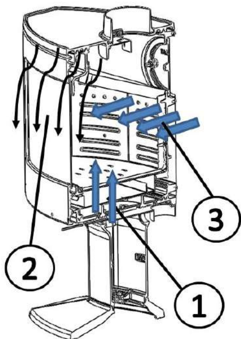
Figura n°16 - Entrata dell'aria di combustione
